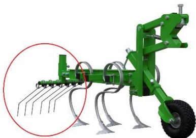
BOM470/2 ET avec dents et étrille
