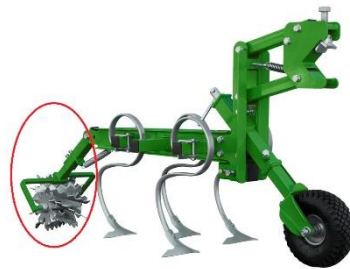
BOM470/2 BA avec dents et rouleau barre
