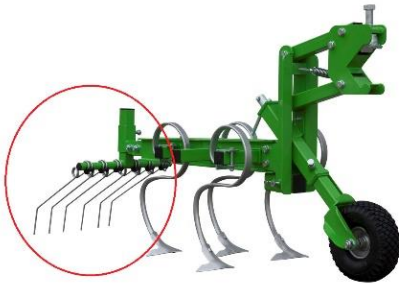
BOM470 ET avec dents et étrille
