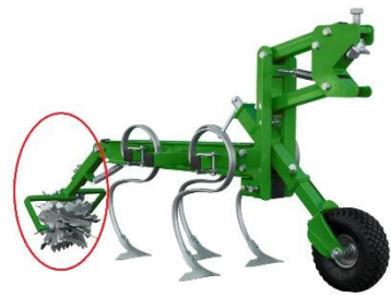
BOM470 BA avec dents et rouleau barre
