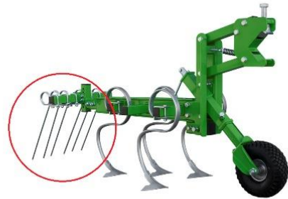
BOM470 ETR avec dents et étrille racleuse
